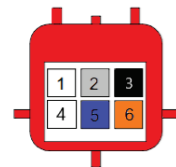
Pinout connettore OBD per Moto (ISO19689:2016) 6 pin vista lato inserzione contatti
